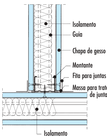
C Conexão em T Transmissão acústica por flancos R_{L,w,R} = 53 \text{ dB}
