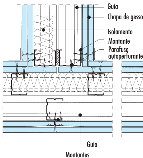
C Conexão em T Transmissão acústica por flancos R_{Lw,R} = 57 dB
