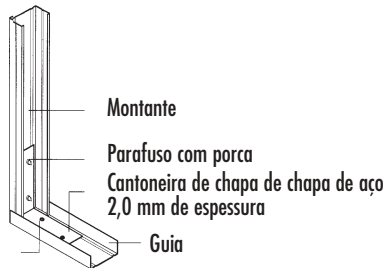
Detalhe A - Fixação dos montantes da porta
