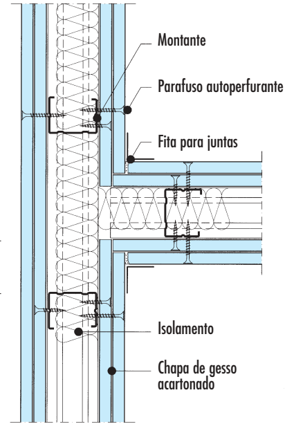
Conexão em T
