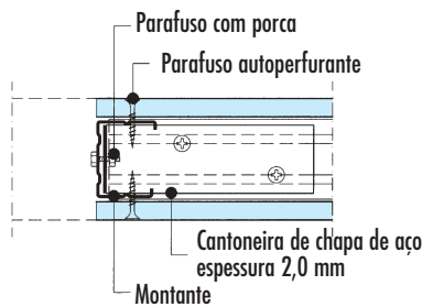
E Configuração da porta
