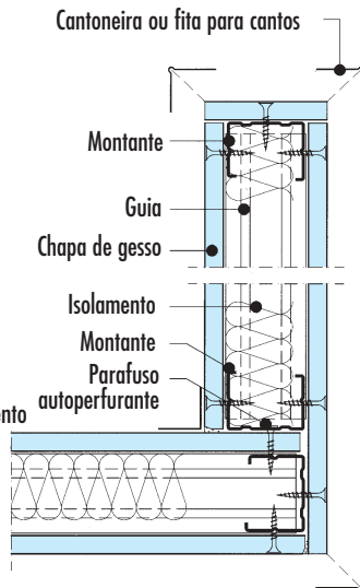
D Conexão de canto
