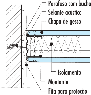
A Encontro com parede maciça
