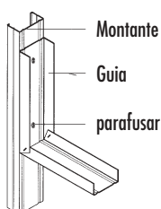
Detalhe B - Estrutura da armação da porta com guia
