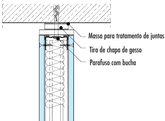
Encontro rígido
